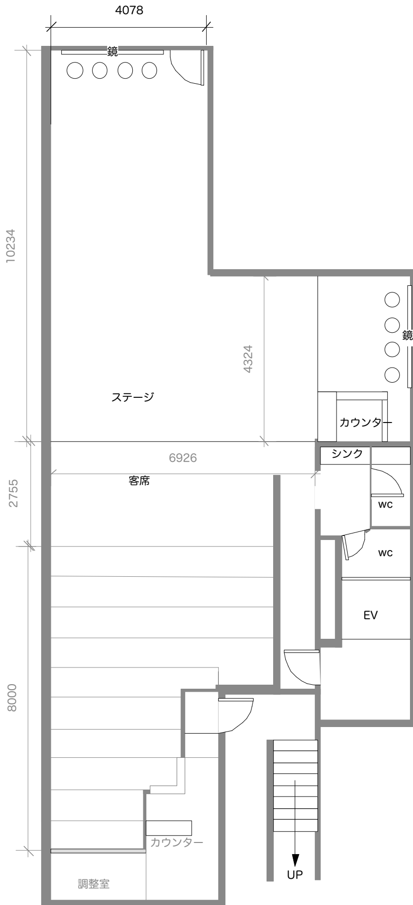
四谷3丁目ドリームシアター 全体平面図1/100 :A3
